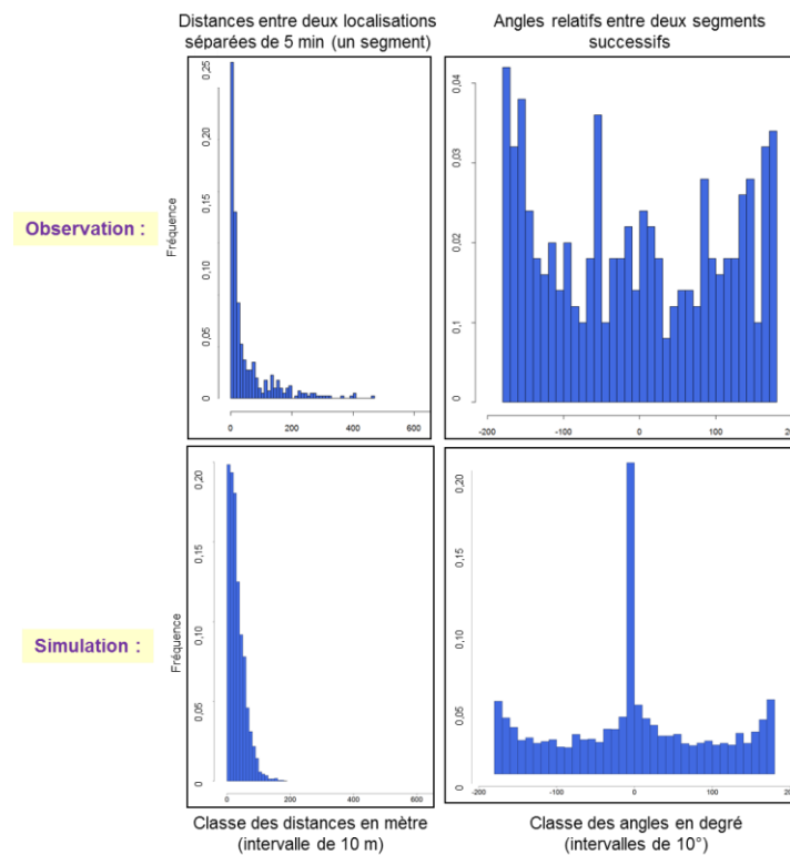
Figure IV.32. Comparaison des distributions des distances et celles d'angles relatifs entre les observations sur un renard et les résultats de 30 simulations par un agent sur le même site d'étude en milieu urbanisé, sur des intervalles de temps de 5 minutes.
