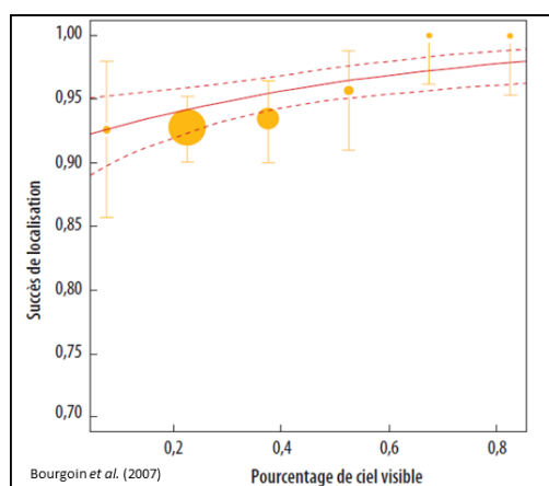
Figure I.16. Relation entre la proportion de ciel visible et le succès de localisation par des colliers GPS (marque Lotek 3300S). Résultats à partir du suivi de 13 femelles de mouflon dans le massif du Caroux-Espinouse dans l'Hérault entre 2003 et 2006. Le rayon des cercles est proportionnel au nombre de positions enregistrées. Les valeurs prédites par un modèle théorique suivent la ligne continue, les lignes pointillées sont les quantiles de 2,5 % et 97,5 % (Bourgoin et al. , 2007). Les faibles pourcentages de ciel visible entraînent une mauvaise réception des signaux des satellites par le collier GPS, ce qui diminue la précision des enregistrements.
