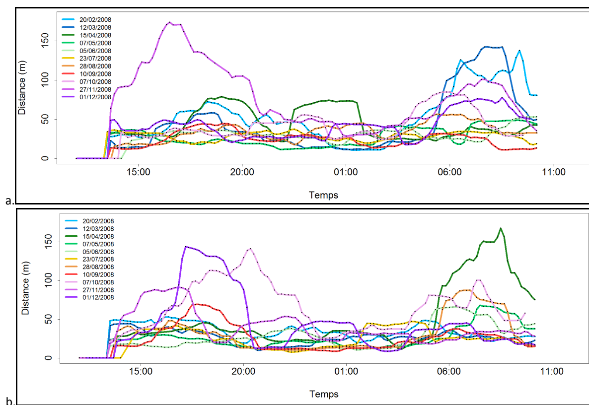
Figure III.14. Valeurs de distances calculées à partir de la méthode des moyennes mobiles sur 9 valeurs en fonction de l'heure, à partir des distances parcourues estimées dans des intervalles de temps de 10 minutes. Représentation d'une même période de 24 h par mois entre février et décembre 2008 pour 2 chevrettes femelles adultes dans le canton d'Aurignac (a et b). Une couleur correspond à une date. Les domaines vitaux de ces 2 chevrettes sont composés principalement de cultures et de petites zones boisées.
