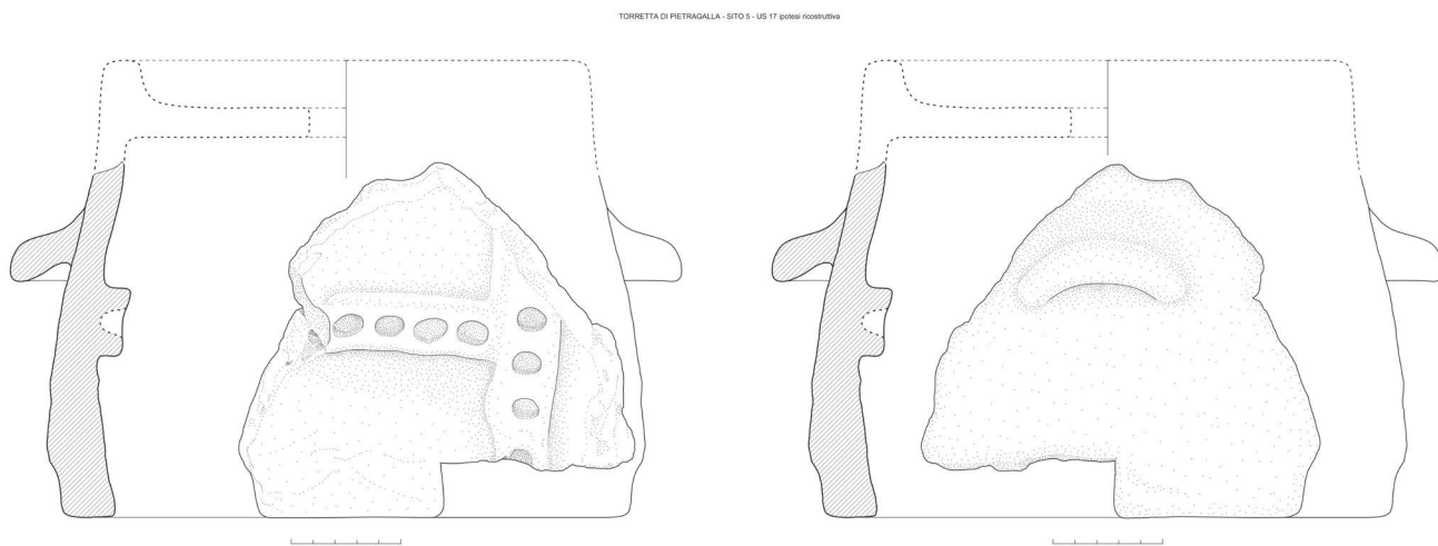
Fig. 14 - Fornello ad impasto da Monte Solario (ricostruzione D. Bruscella).
