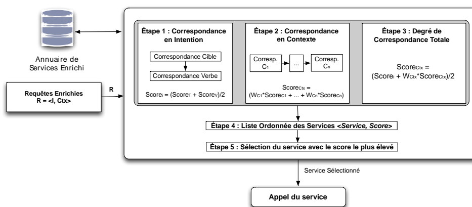
FIG. 1. Schéma du mécanisme de découverte de services guidé par l'Intention et le Contexte
