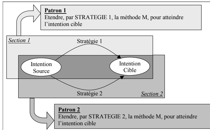
Figure 5: Equivalence entre le concept de section et celui de patron
