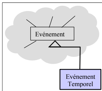
Figure 16: Exemple d'insertion par le biais d'un lien d'héritage (Cas 1)
