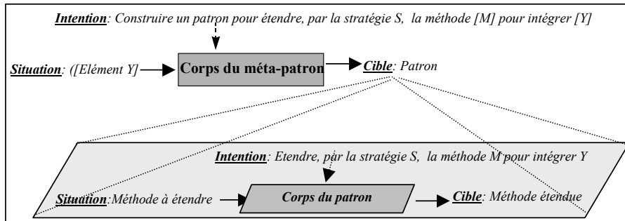
Figure 12. Interface d'un méta-patron
