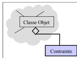
Figure 18: Exemple d'insertion par le biais d'un lien de composition (Cas 1)
