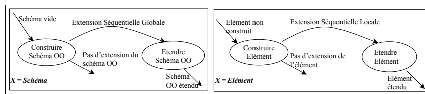
Figure 21. Principes des extensions globales et locales
