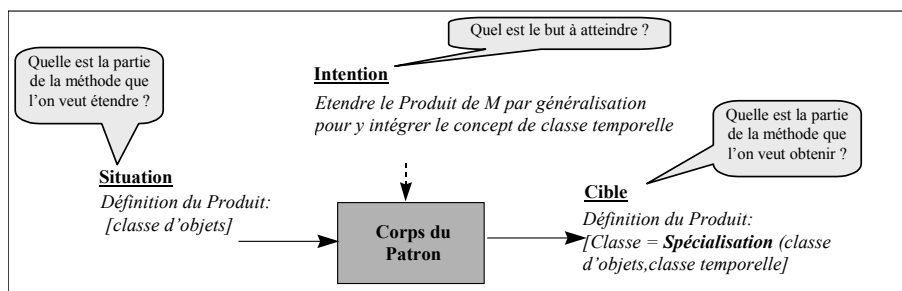
Figure 2: Partie Interface d'un patron
