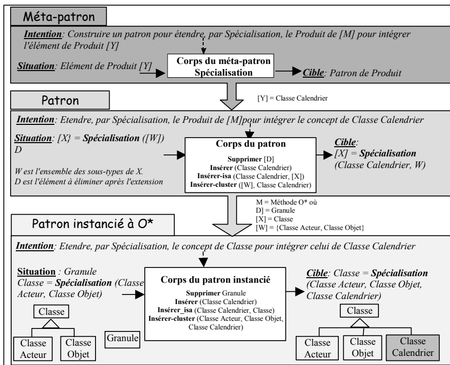
Figure 14. Exemple d'utilisation d'un méta-patron
