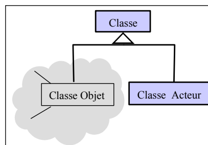
Figure 17: Exemple d'insertion par le biais d'un lien d'héritage (Cas 2)
