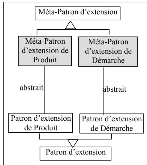
Figure 13: Typologie des méta patrons d'extension de méthodes
