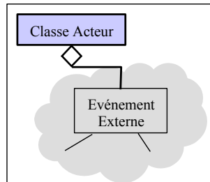
Figure 19: Exemple d'insertion par le biais d'un lien de composition (Cas 2)
