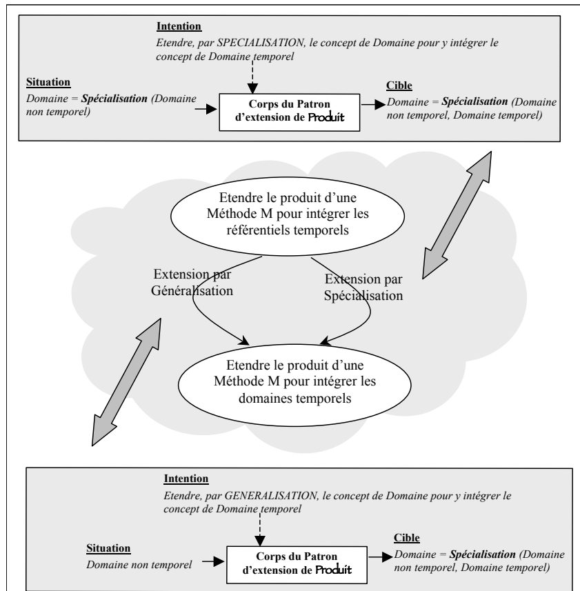
Figure 6: Exemple de Patrons organisés par une carte d'extension
